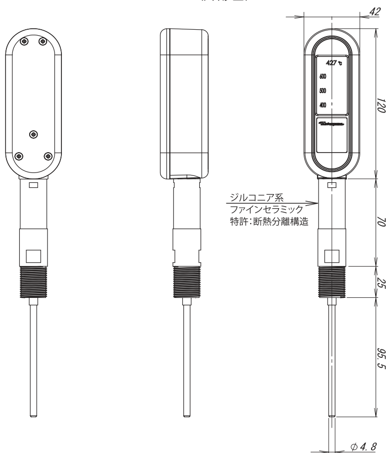
（外形図）
